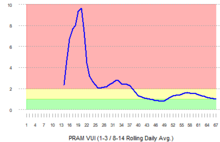
Nebraska PRAM Ventilator Use Index (VUI)
