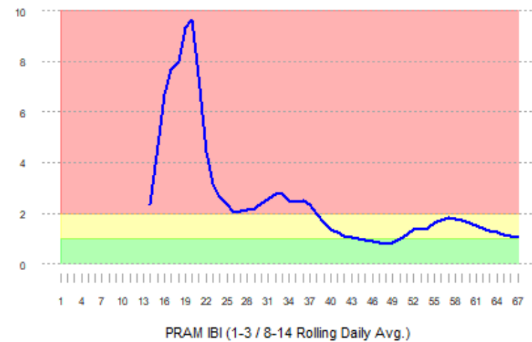
Nebraska PRAM ICU Beds Index (IBI)
